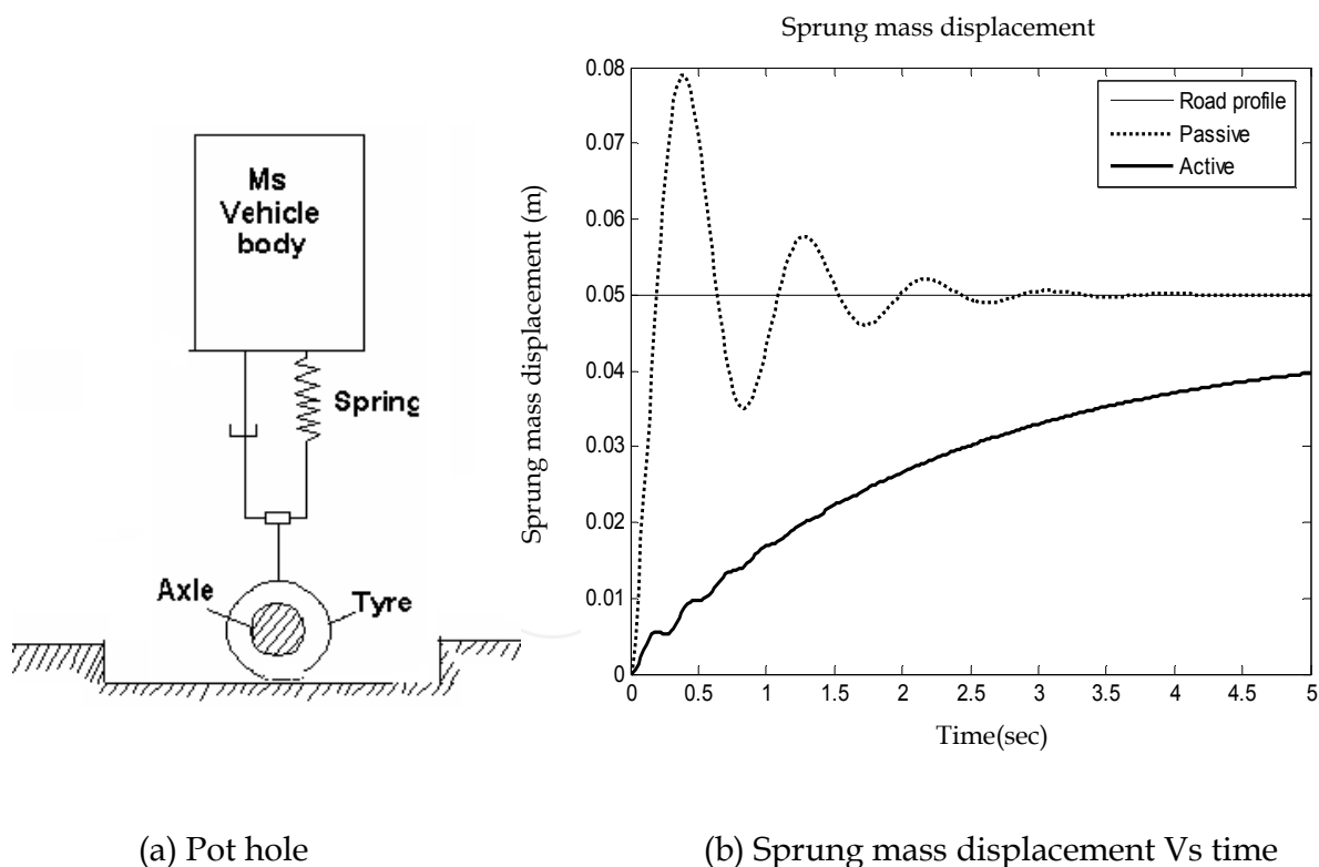
Fig. 23. Sprung mass displacement (Pot hole)
