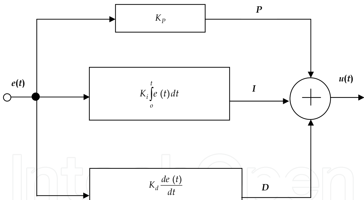
Fig. 4. PID controller
