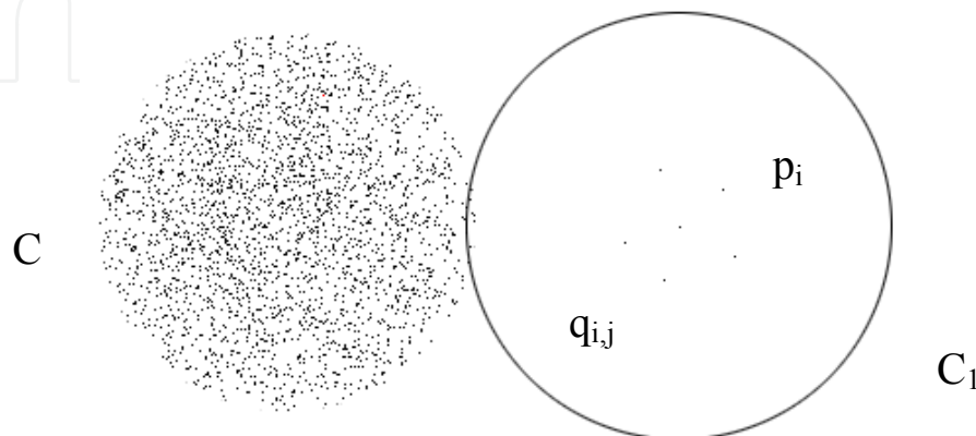
Fig. 6. 2-d Dataset
