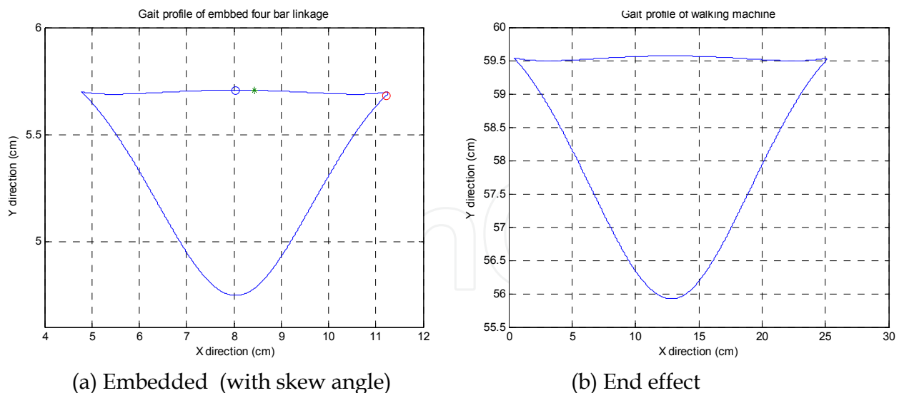
Fig. 6. Gait profile.
