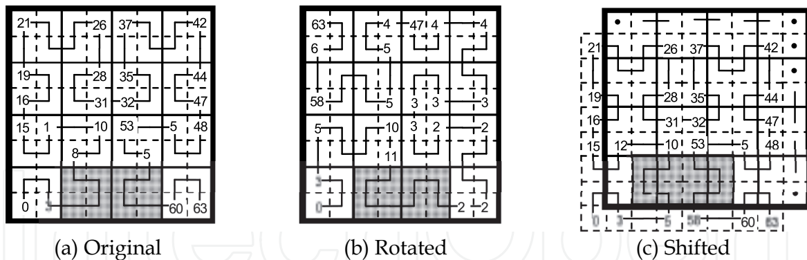
Fig. 1. Range Query A.
