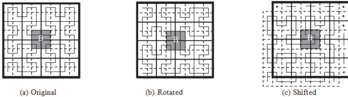
Fig. 3. Range query B.
