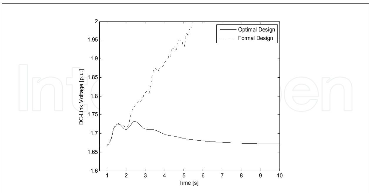
Fig. 19. DC-Link Voltage
