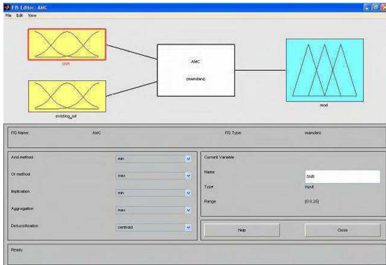
Fig. 11. FIS system
