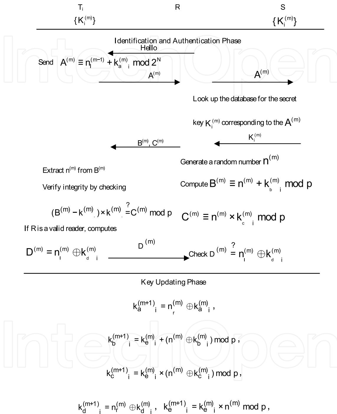
Fig. 1. The UCS-RFID protocol.
